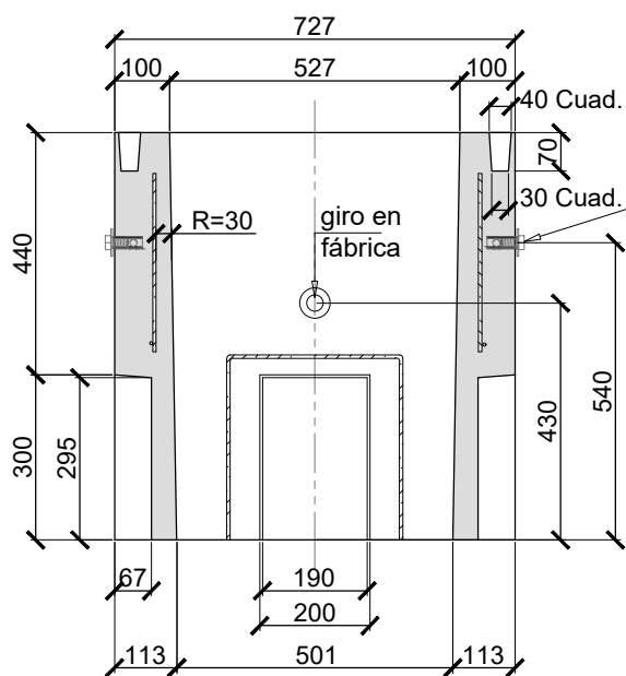
SECCIÓN A-A
