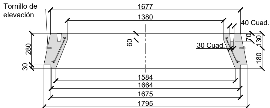
SECCIÓN A-A
