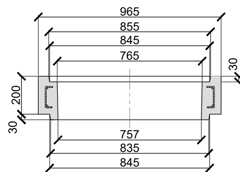
SECCIÓN B-B
