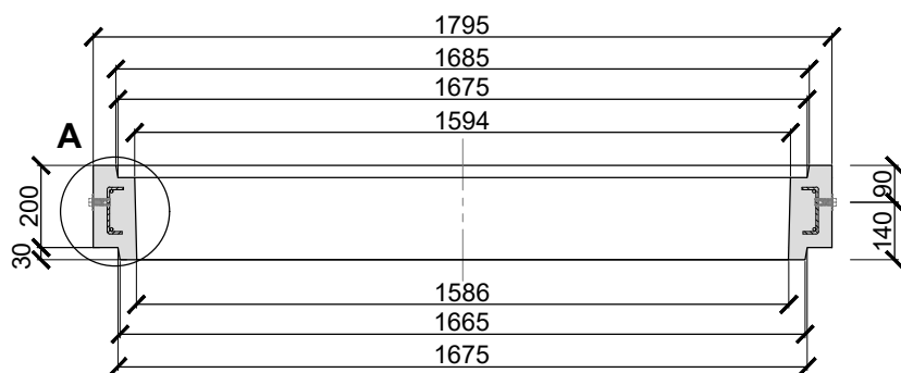
SECCIÓN A-A
