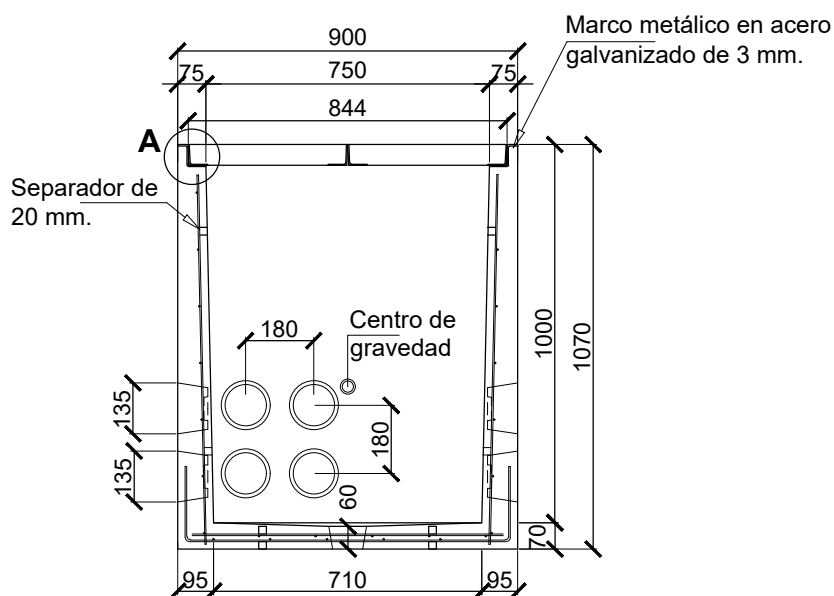
DETALLE A
