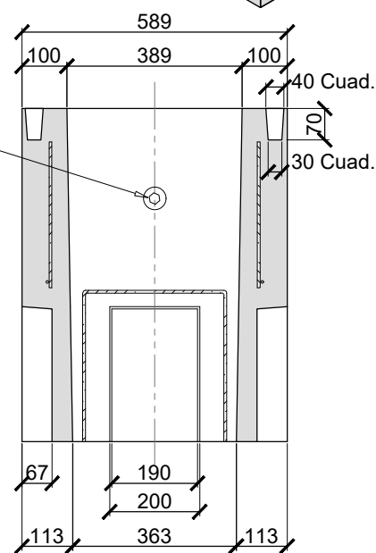
SECCIÓN B-B
