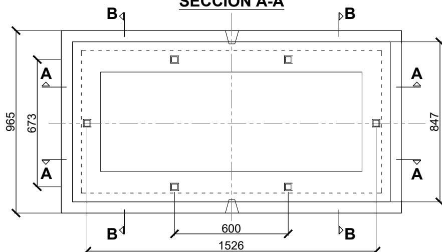
SECCIÓN A-A
