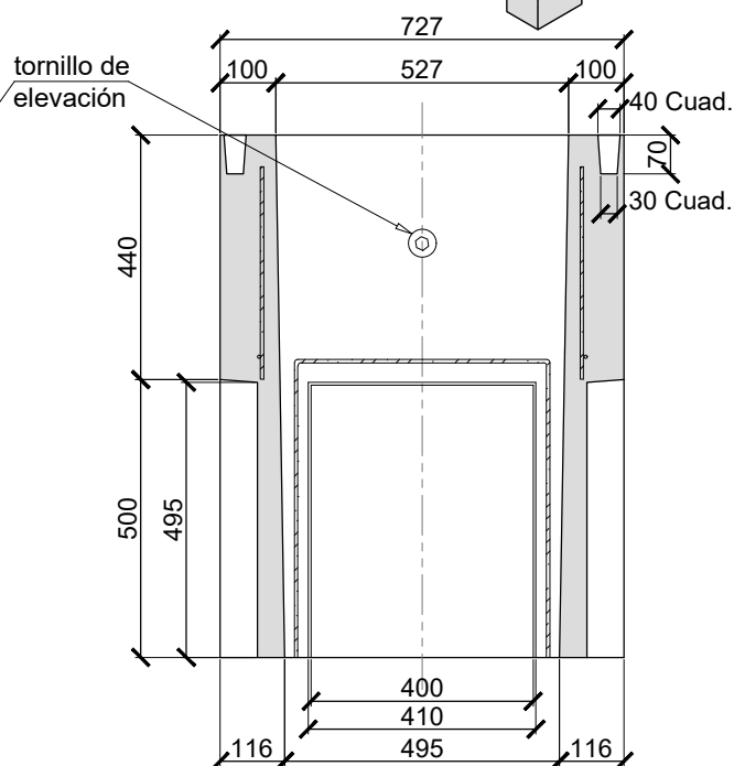
SECCIÓN B-B
