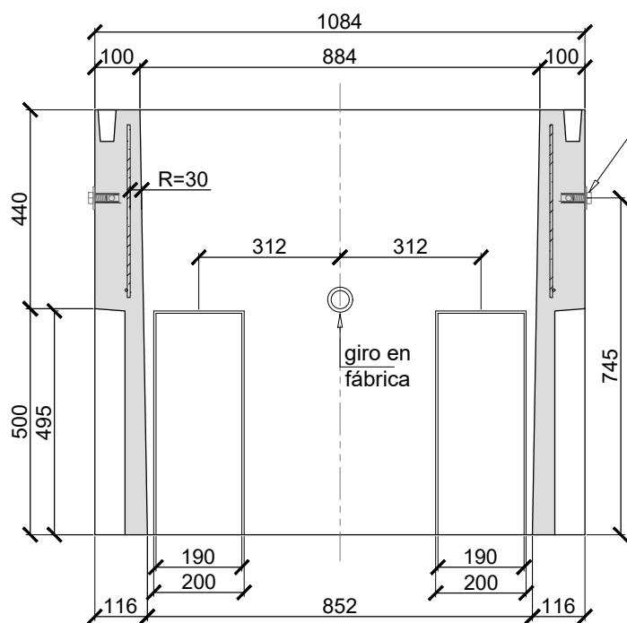
SECCIÓN A-A
