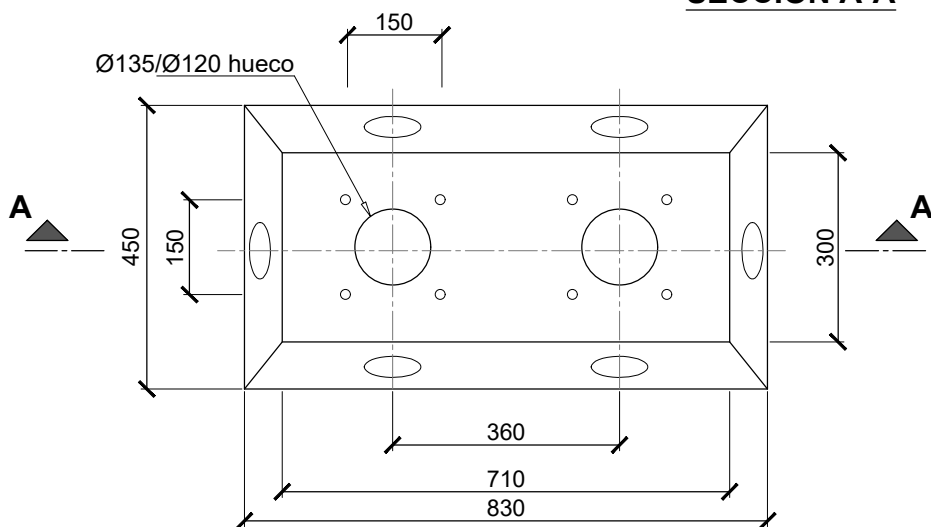
PLANTA
