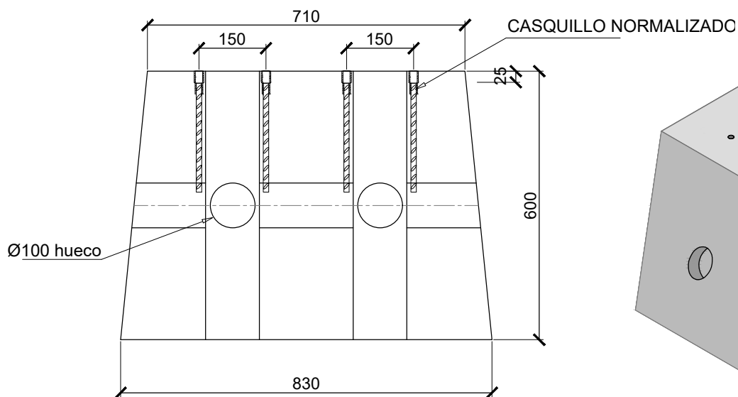
SECCIÓN A-A
